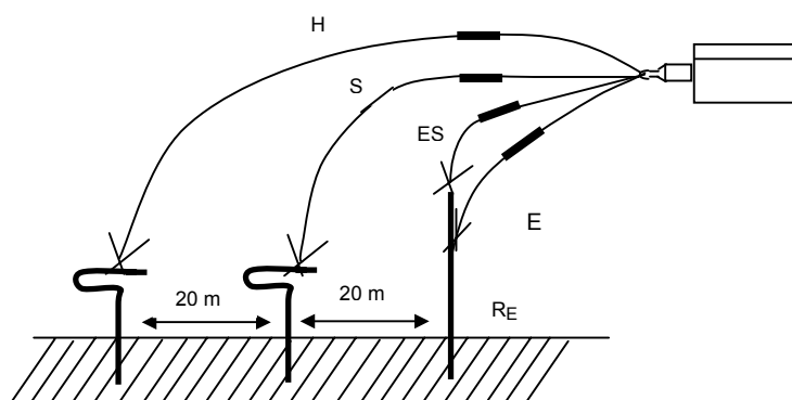
Figura 2. Medida de la resistencia de puesta a tierra R_E .
