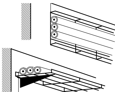
Figura C. Instalación de cables sobre bandejas de rejilla (pueden utilizarse también bandejas ciegas, perforadas o bandejas de escalera)
