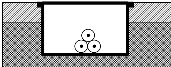
Figura A: Ejemplo de instalación de conductores unipolares aislados en canal protectora empotrada en suelo o pared
